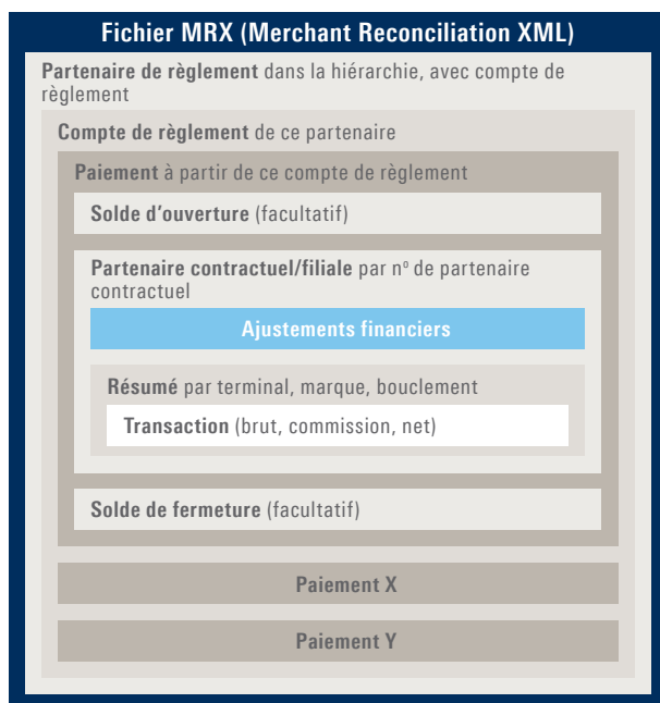
Structure schématique d'un fichier MRX.
